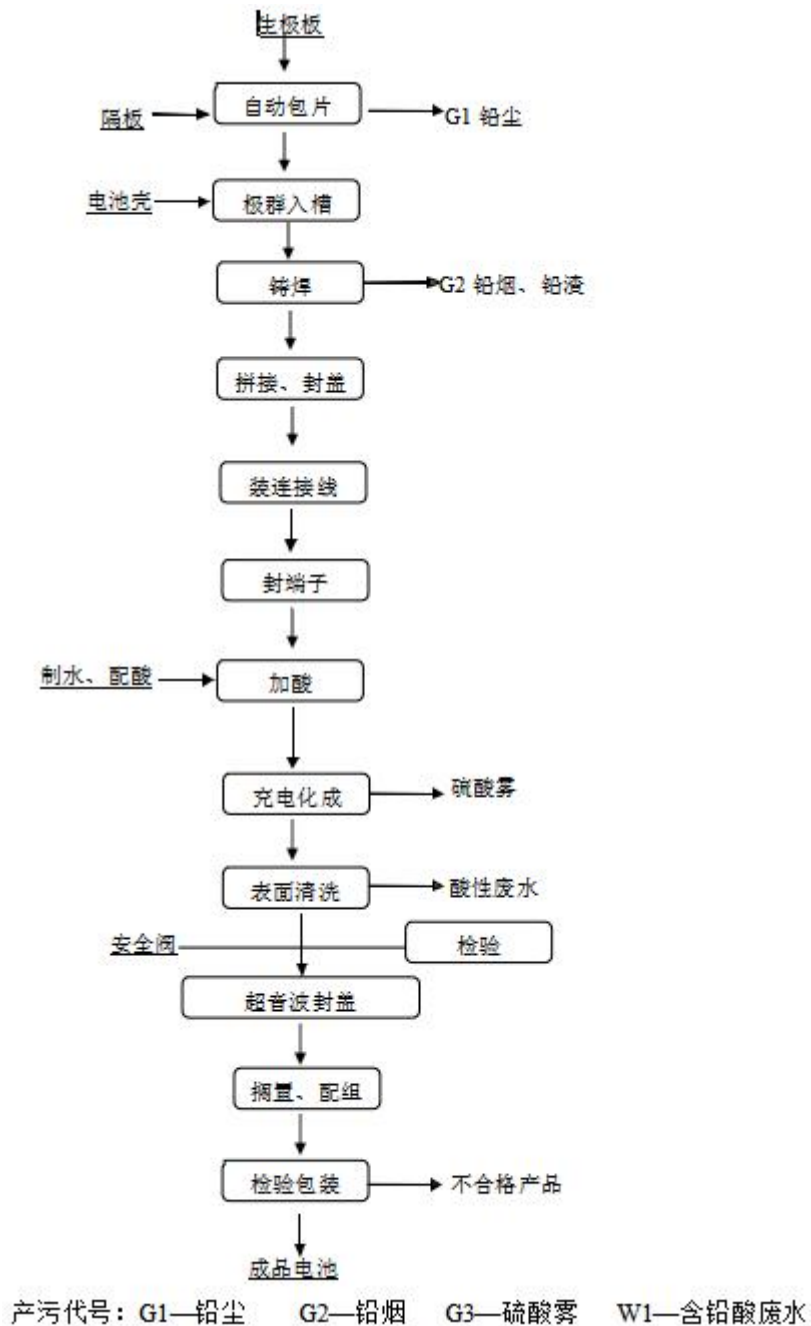
图3.2-2 蓄电池装配生产工艺流程及产污环节图
