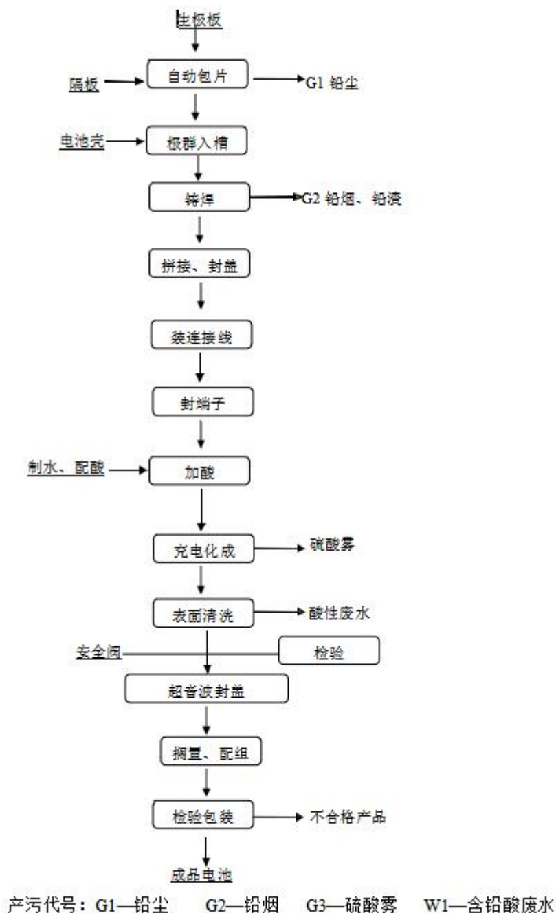
图2.2-2 蓄電池裝配生產工藝流程及產污環節圖
